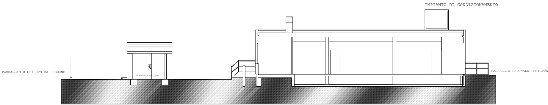
SEZIONE B-B
